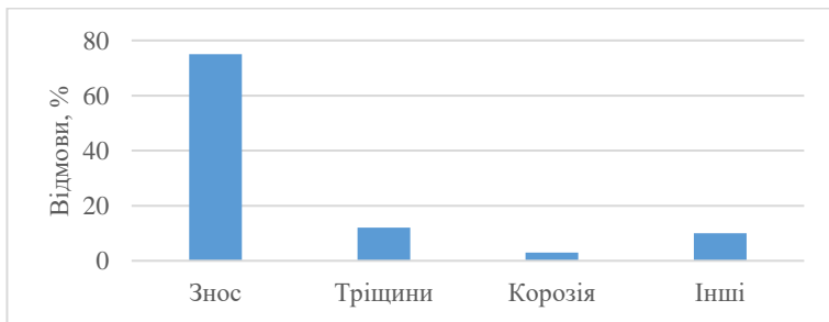
Рис. 2. Відмови валів насосного агрегату НЖФ-150
