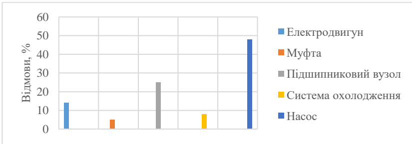
Рис. 1. Відмови насосного агрегату НЖФ - 150
